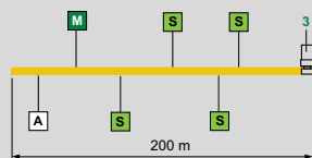
M Module maître S Interface ou composant A Alimentation AS-Interface 3 Extension de ligne TCSAAR011M 4 Répéteur ASI RPT01
