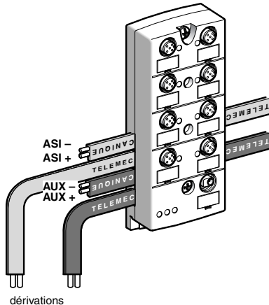
Exemple de dérivation sur module 8 voies
