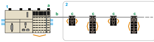
Ilots d'entrées/sorties distribuées IP 67 Entrées/sorties
