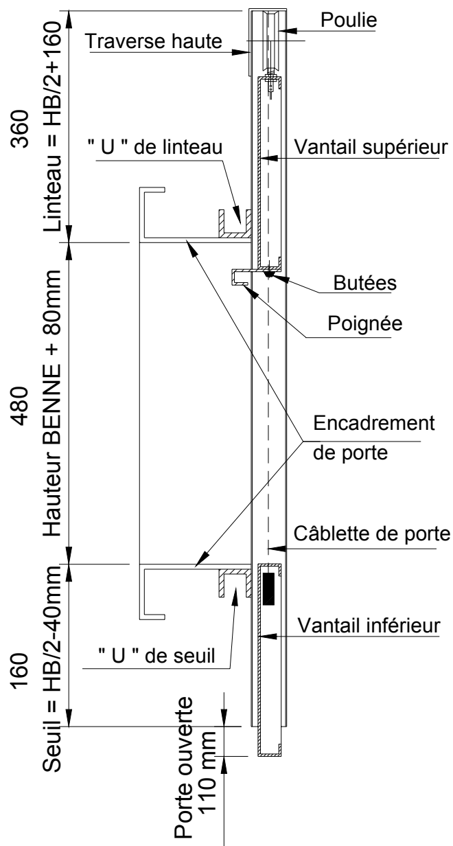
Coupe de la porte
