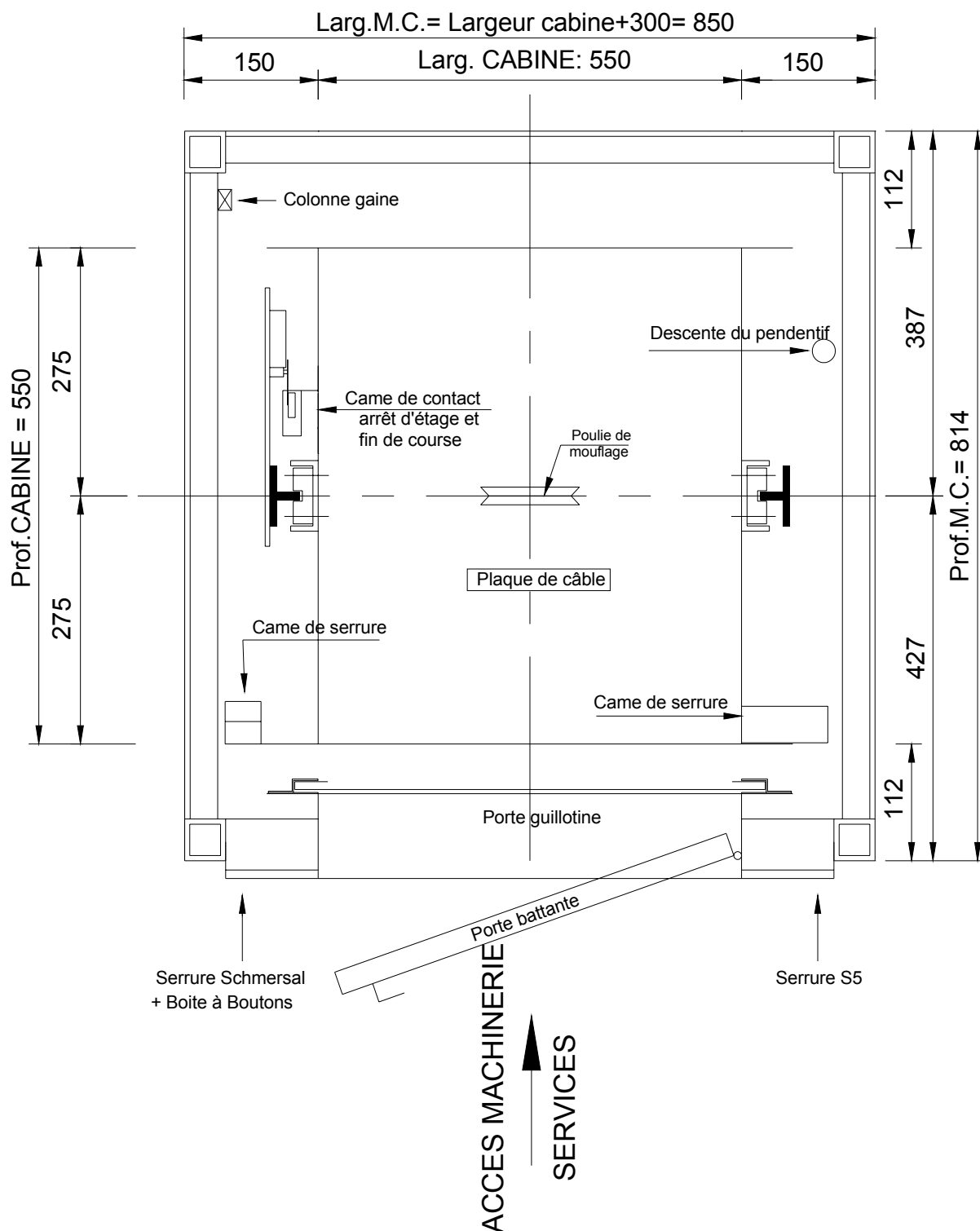
Vue de la cabine - Poulie - Guide - Came
