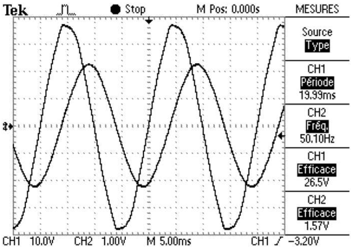
Circuit RL - Mesure du déphasage
