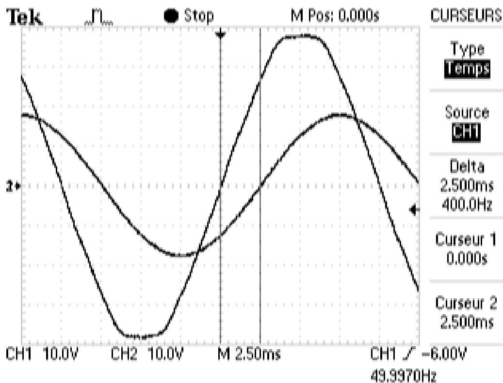
Mesure du déphasage phi de i(t)/u(t)
