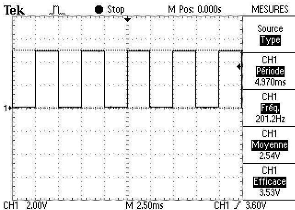
Signal Carré Symétrique et Positif
