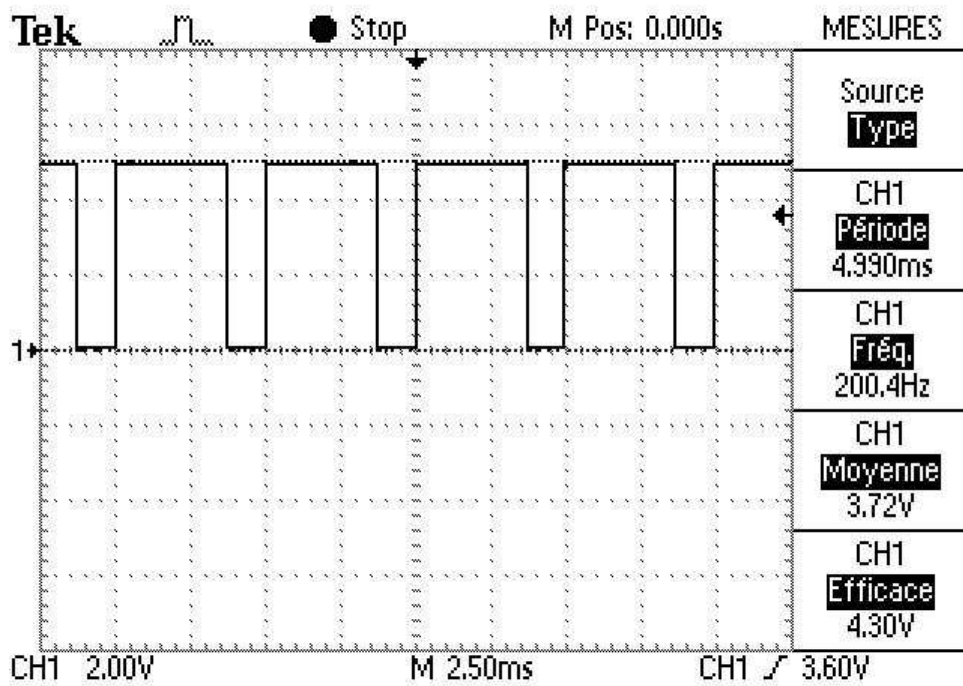
Signal Carré Non Symétrique et Positif
