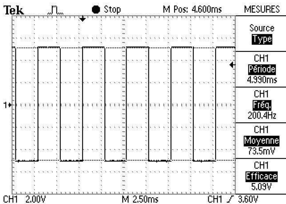
Signal Carré Symétrique
