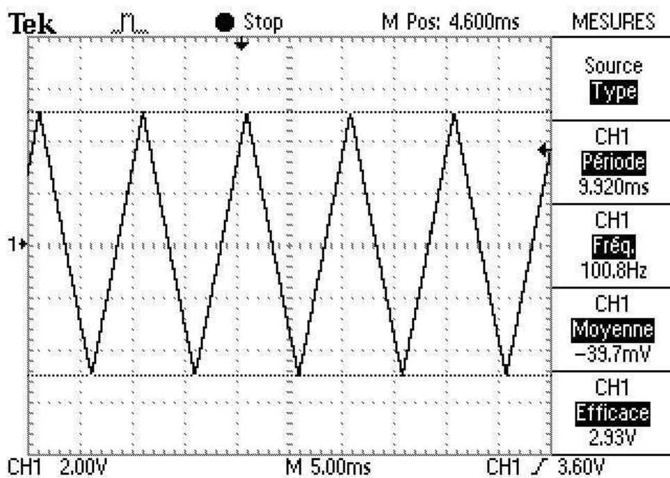
Signal Triangle Symétrique
