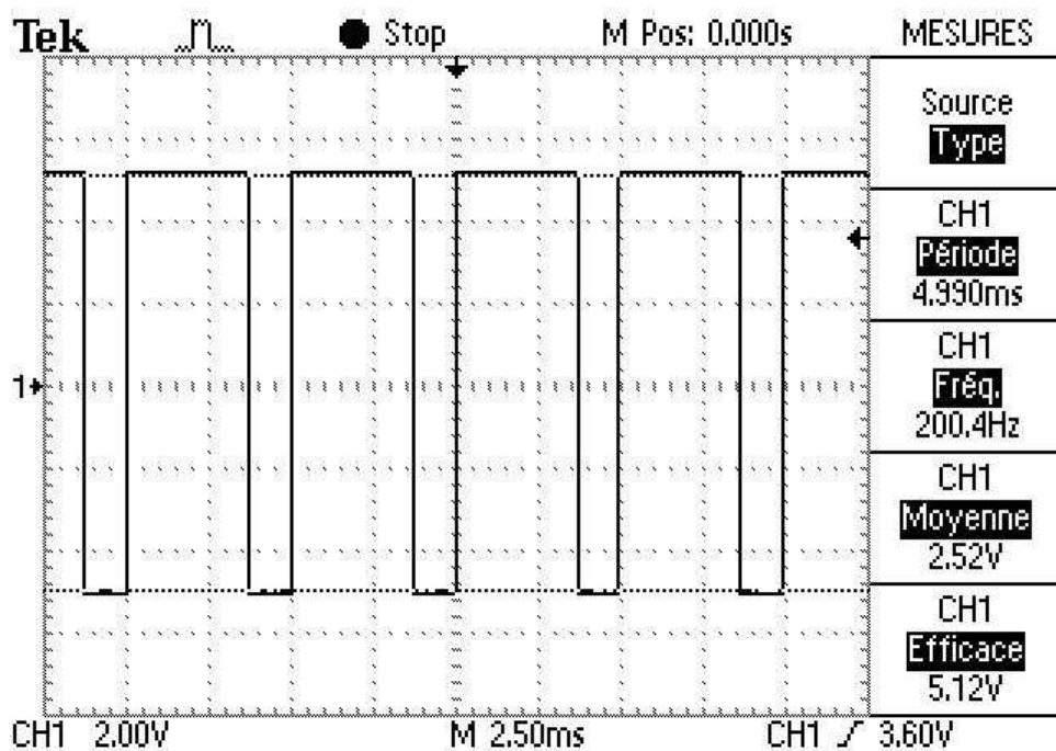
Signal Carré Non Symétrique
